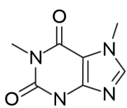
1. Caffeine
