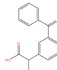
4. Ketoprofen
