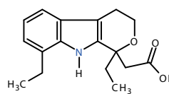
Etodolac
